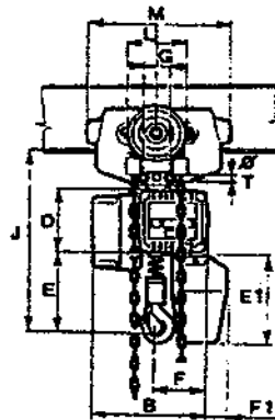
4C PARANCO CON CARRELLO A CATENA HOIST WITH MECHANICALLY-OPERATED CHAIN TROLLEY PALAN AVEC CHARIOT MECANIQUE À CHAÎNE E-ZUG MIT KETTENKATZE
