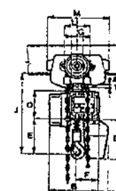
4C PARANCO CON CARRELLLO A CATENA PALAN AVEC CHARIOT MECANIQUE A CHAÎNE
