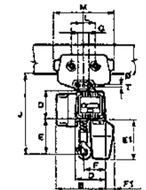
2S PARANCO CON CARRELLLO A SPINTA PALAN AVEC CHARIOT PAR POUSSEE
