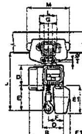
3E PARANCO CON CARRELLLO ELETTRICO PALAN AVEC CHARIOT ELECTRIQUE
