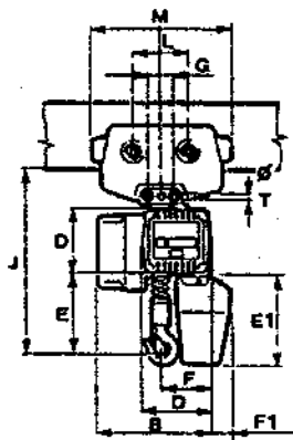
2S PARANCO CON CARRELLO A SPINTA HOIST WITH HAND-PUSHED TROLLEY PALAN AVEC CHARIOT PAR POUSSÉE E-ZUG MIT ANGESCHOBENER KATZE
