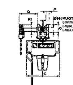
HOIST WITH MECHANICALLY OPERATED CHAIN TROLLEY E-ZUG MIT KETTENKATZE
