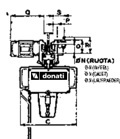
HOIST WITH ELECTRIC TROLLEY E-ZUG MIT ELEKTRISCHER KATZE
