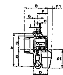
1F PARANCO IN ESECUZIONE FISSA PALAN EN EXECUTION FIXE
